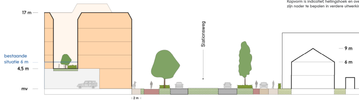
Profiel D-D'
